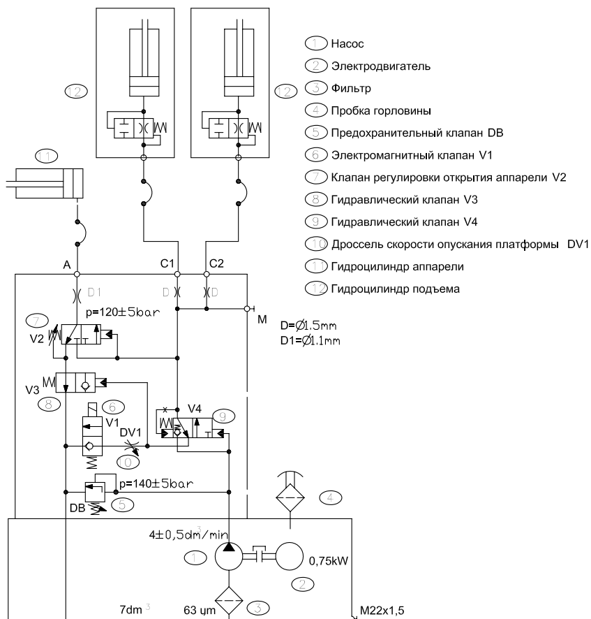
Рис. 1. Гидравлическая схема
